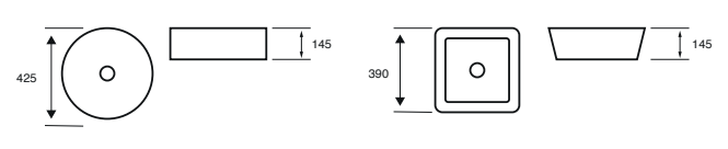
LOIS SQUARE 390MM
